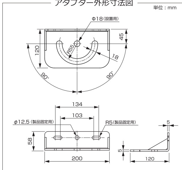
アダプター外形寸法図
