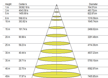
照度図
