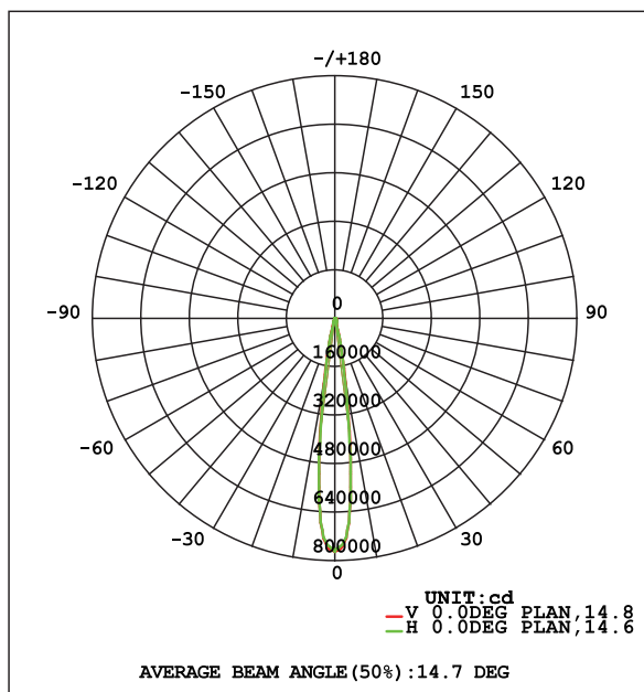
配光曲線
