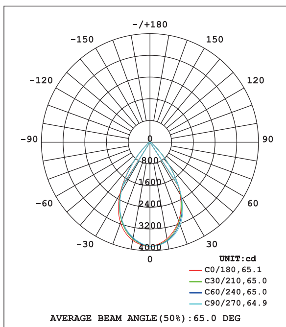
配光曲線
